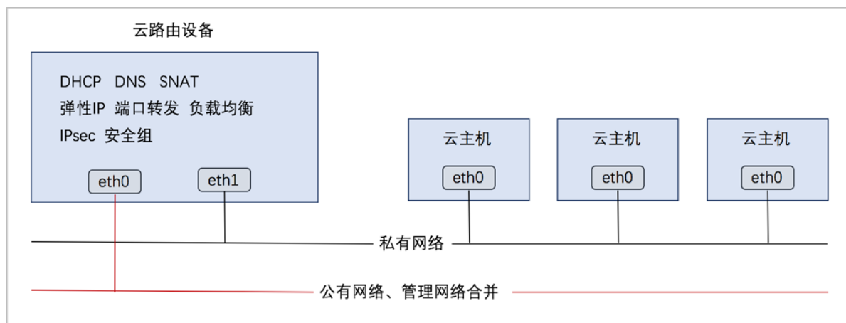
图 1: 部署方式-1
